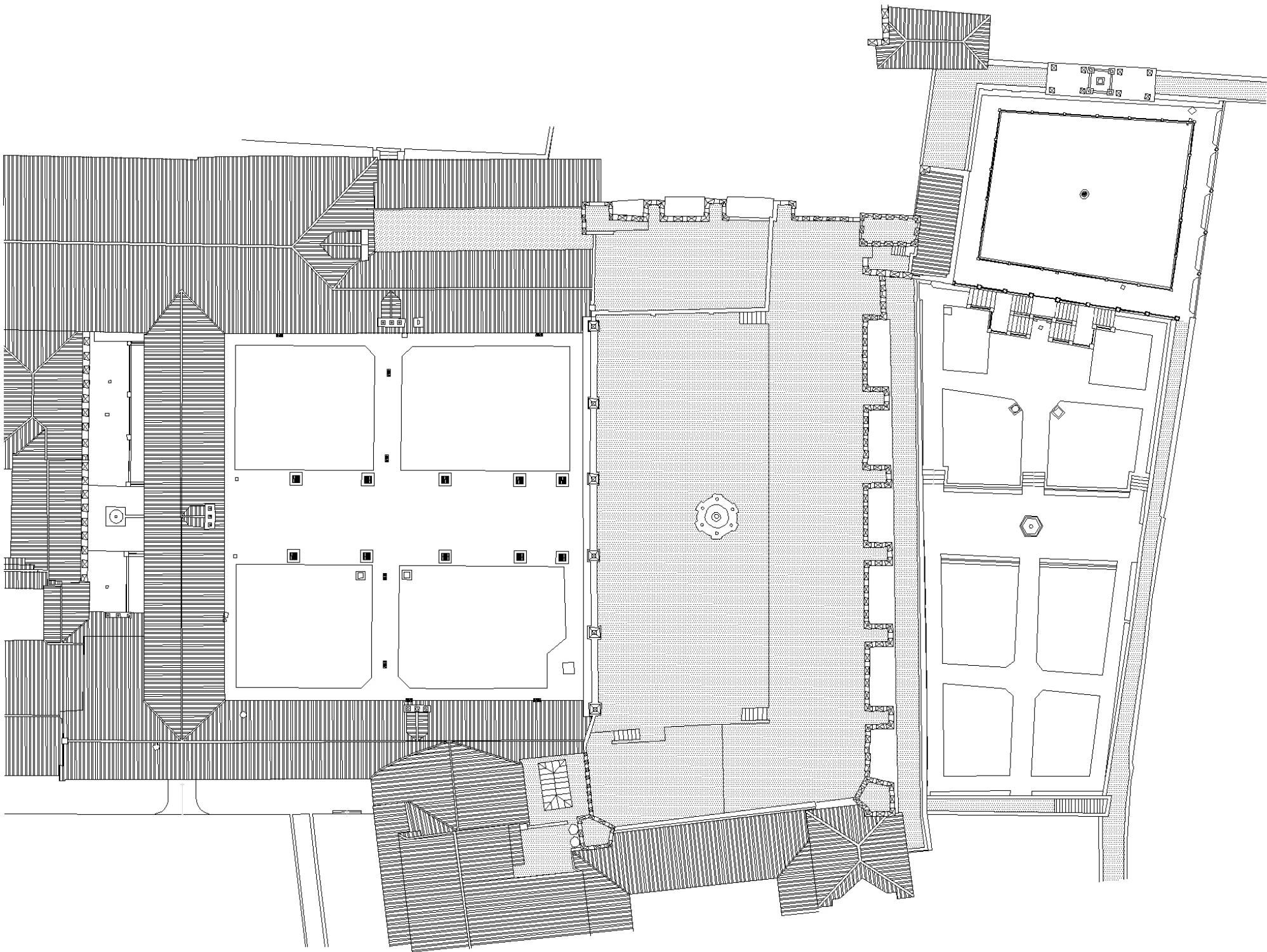
ALCAZAR DE SEVILLA. PLANTA DE CUBIERTAS. PATIO DE CRUCERO Y PALACIO GÓTICO. ESCUELA DE ESTUDIOS ÁRABES, C.S.I.C. A.ALMAGRO/ arg. LZUNIGA/ arg.tec.
